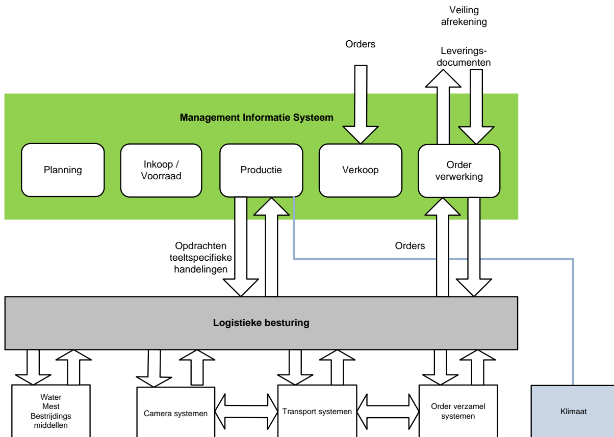
Figuur 14: Het architectuurmodel van Plantform
